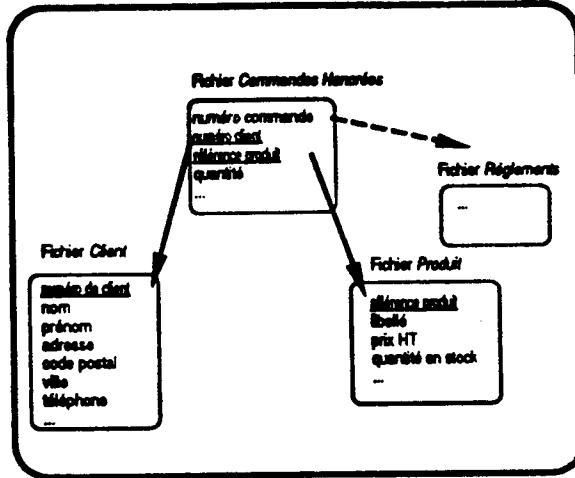
Fig. 2: Les Bases de données relationnelles.
